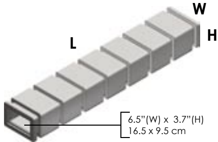
FS120-B 47.2"(L) x 8.7"(W) x 6"(H) 120 x 22 x 15 cm
